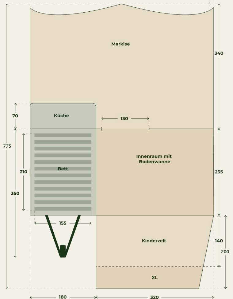
Auf dem obigen Bild ist die Aero MTT (mit Küche) abgebildet
